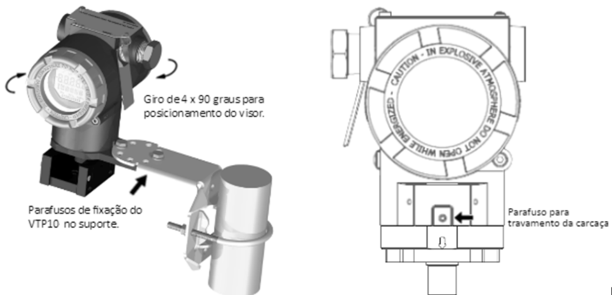
Figura 2.3 – Fixação do VTP10-P no suporte e rotação da carcaça 4 x 90° com travamento.
