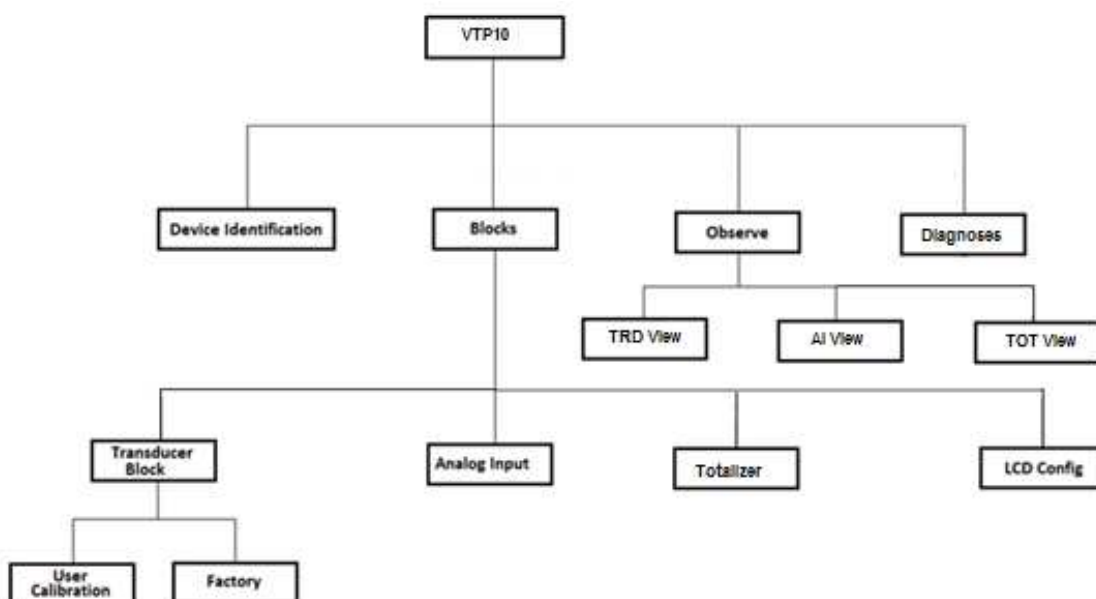
Figura 3.6 – Árvore de programação do VTP10-P.
