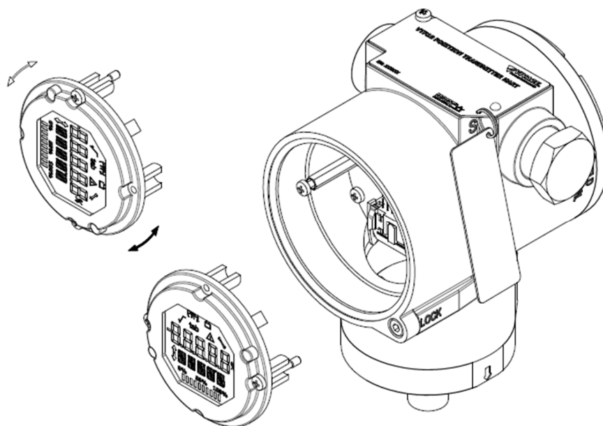
Figura 2.4 – Rotação do display digital LCD 4 x 90°
