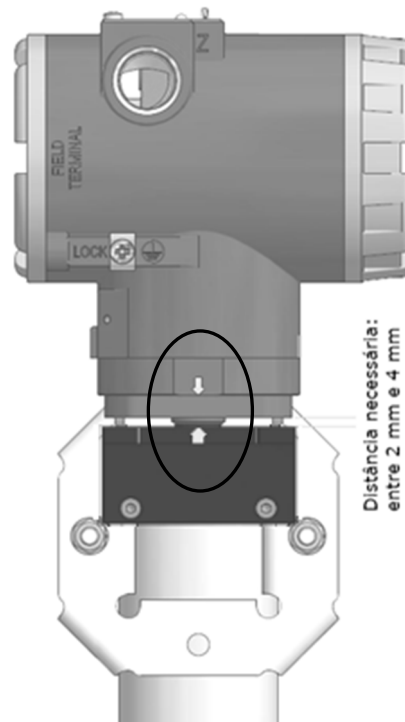
Figura 2.6 – Montagem do VTP10-P em ímã linear.
